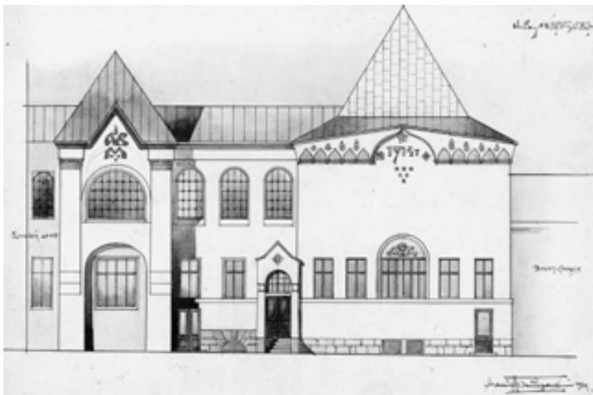
Пристройка к особняку А. Морозова. Проект Архитектор И.Е. Бондаренко
